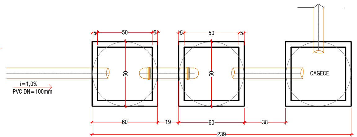
Planta Baixa - Sistema SAO com Filtro Ascendente Esc. - 1:20
