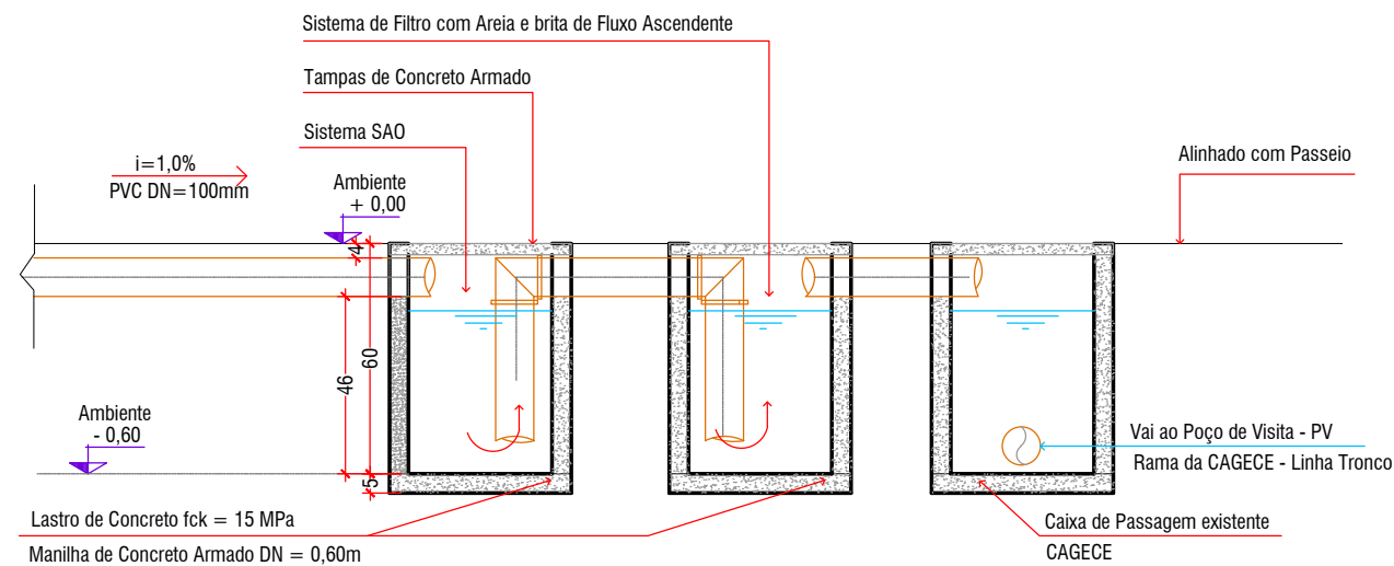
Planta - Corte A-A e Detalhe A Esc. - 1:20
