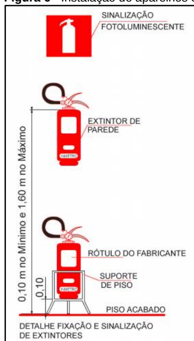
Figura 6 - Instalação de aparelhos extintores.
