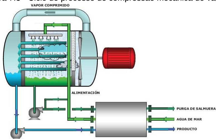
Figura 7.3 - Ciclo do processo de compressão mecânica do vapor
