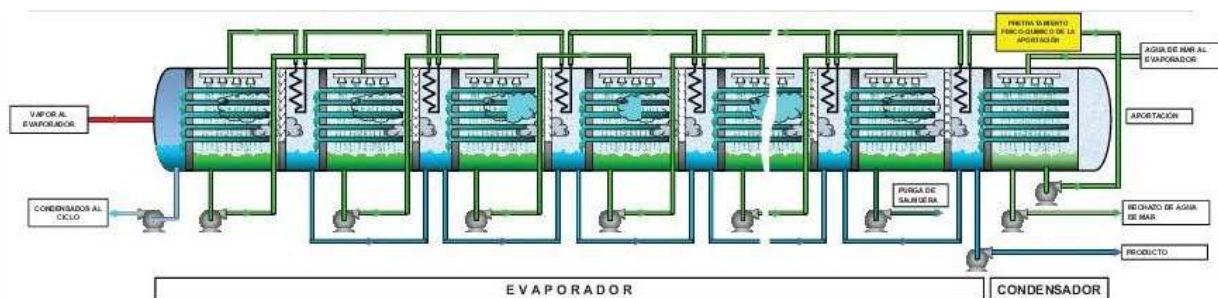
Figura 7.2 - Processo de evaporação multiefeito
