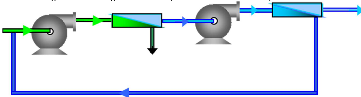
Figura 7.11 - Diagrama de uma planta de OI de duas etapas
