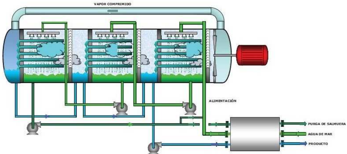
Figura 7.4 - Ciclo do processo de compressão mecânica do vapor (Multietapa)
