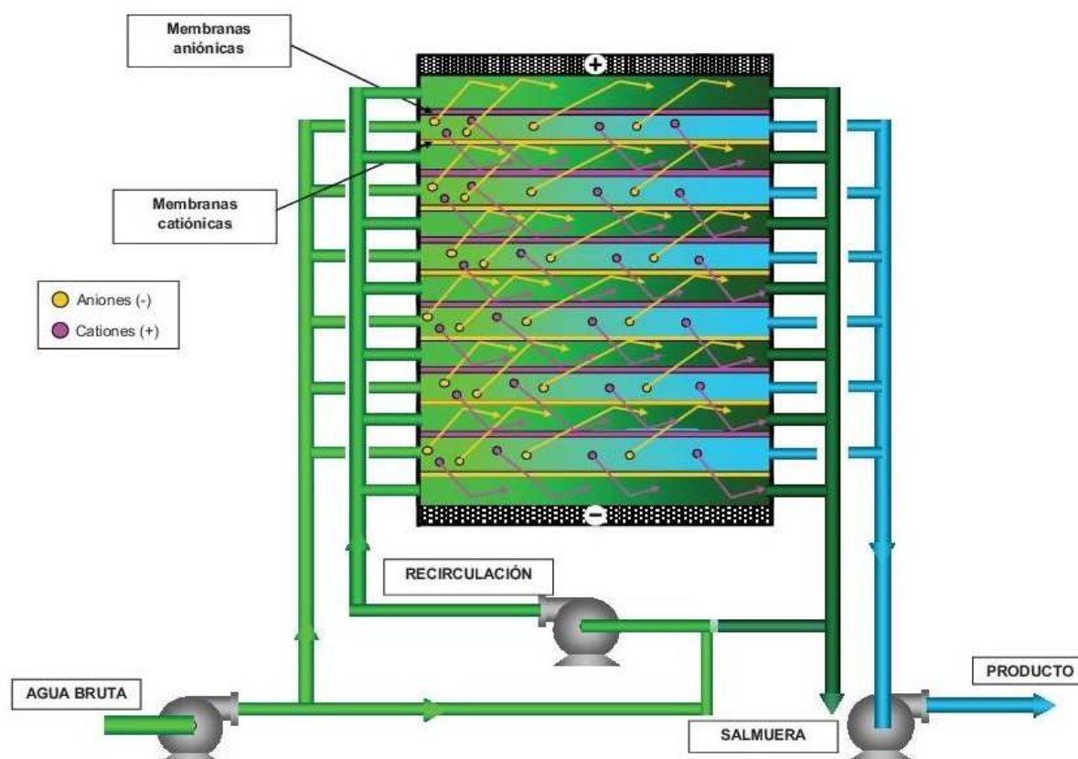
Figura 7.12 - Processo de Eletrodialise
