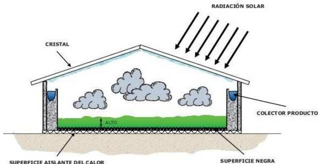
Figura 7.6 - Diagrama da planta de destilação solar direta
