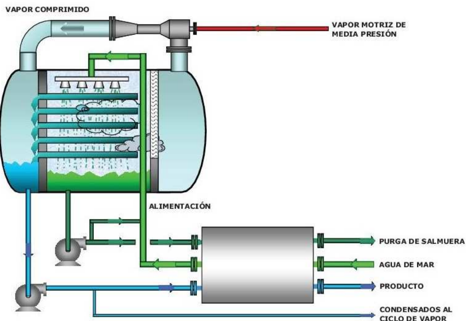
Figura 7.5 - Ciclo de processo de ejeção de compressão de vapor
