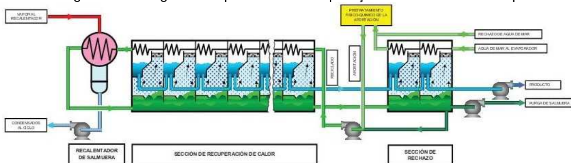
Figura 7.1 - Diagrama do processo de evaporação instantânea Multietapa
