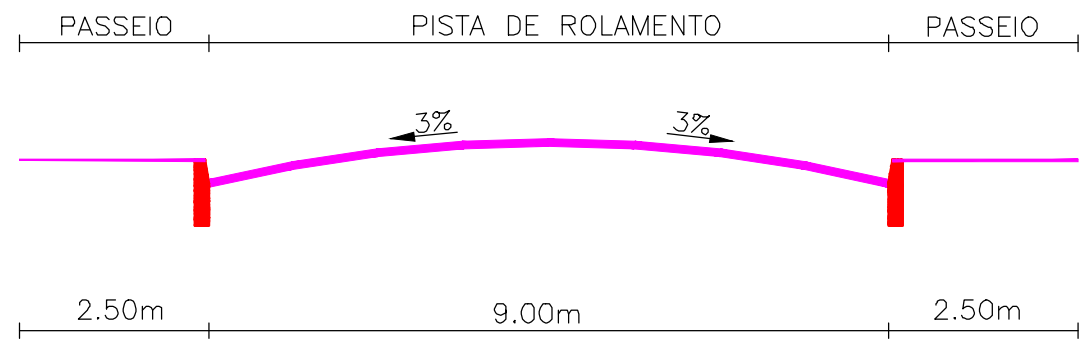
SEÇÃO TRANSVERSAL RUA - ERIBERTO ONOFRE
