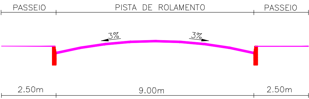
SEÇÃO TRANSVERSAL VIA - LOCAL
