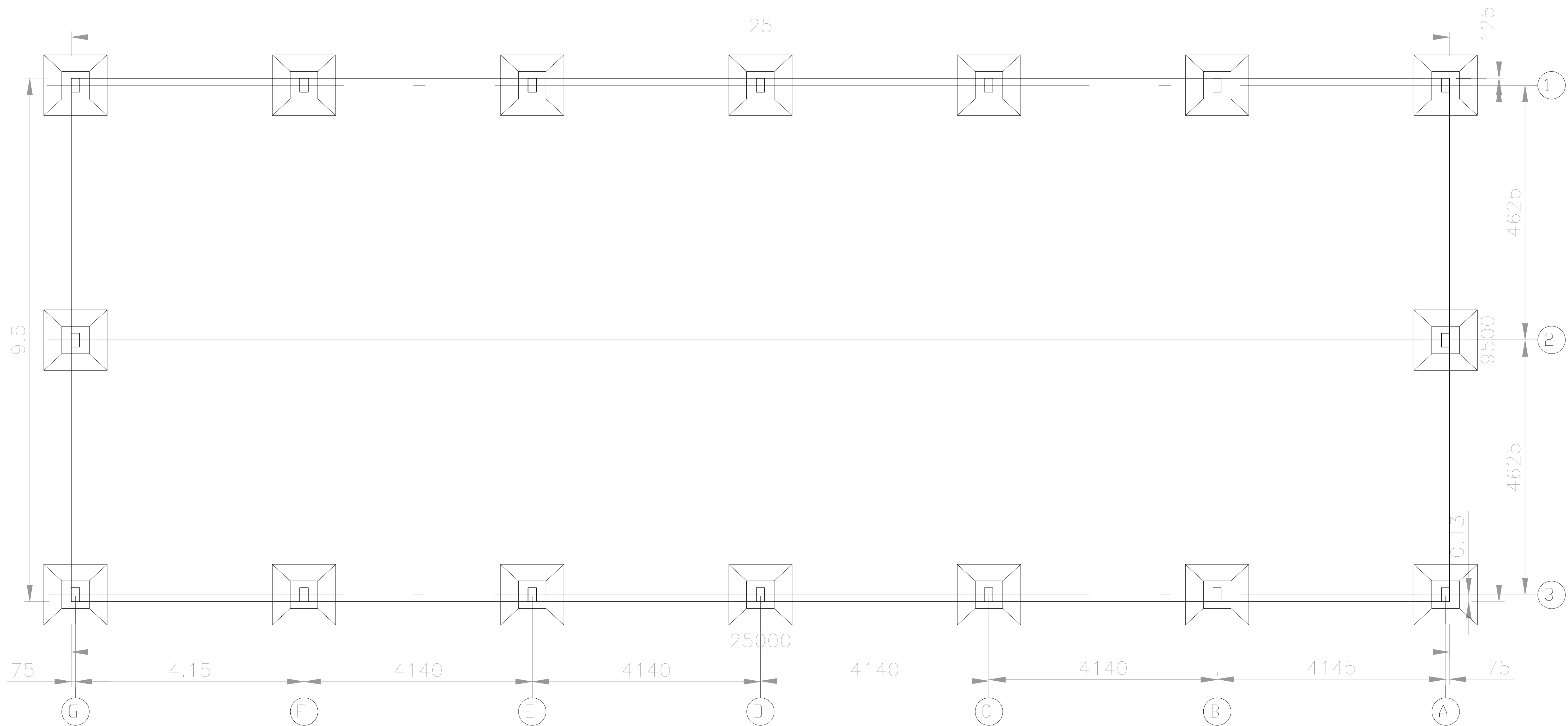
LOCAÇÃO DE SAPATAS ESC.: 1/100
