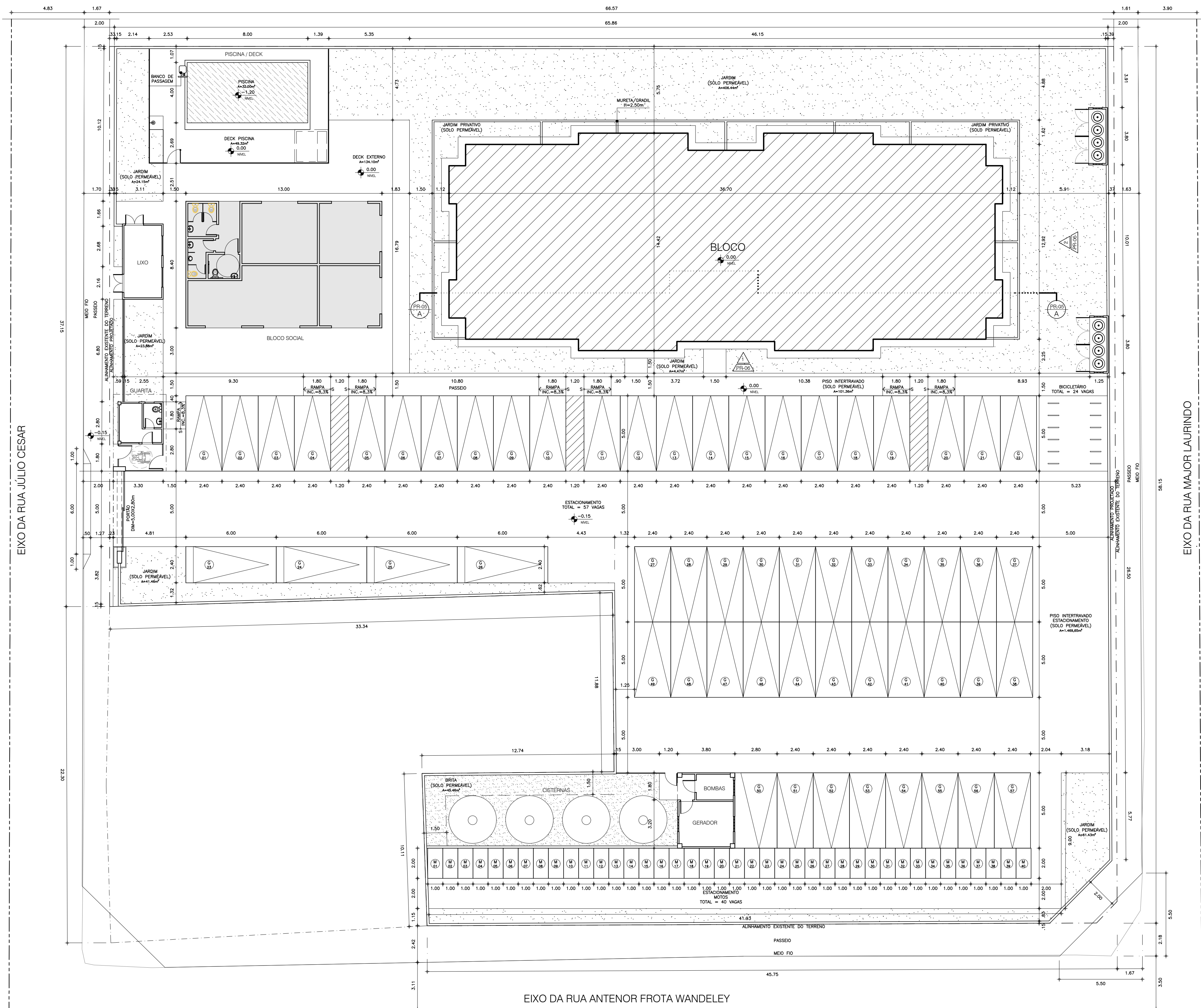
01 PLANTA DE SITUAÇÃO / TÉRREO ESCALA 1/125
