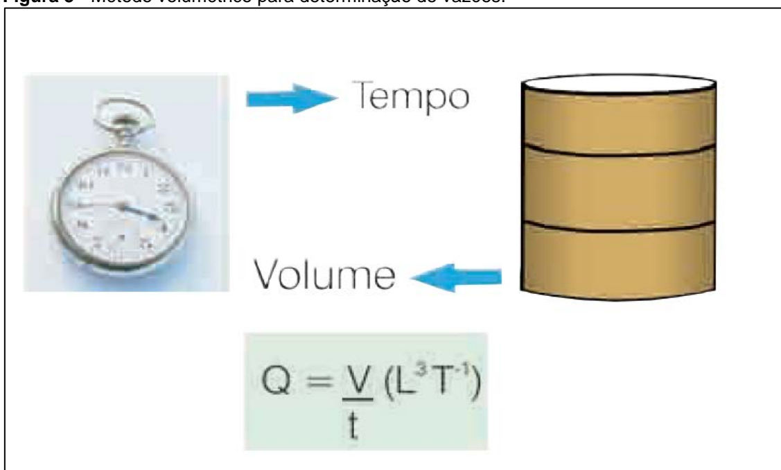
Figura 3 - Método volumétrico para determinação de vazões.
