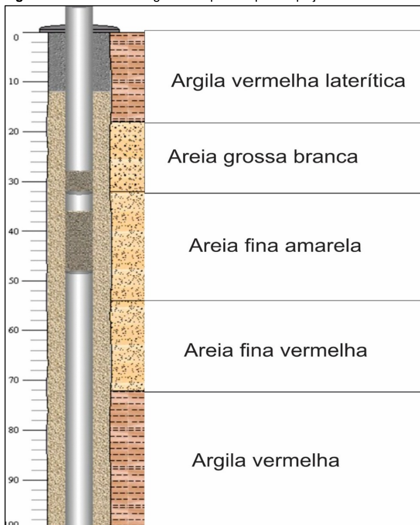
Figura 8 - Perfil litoestratigráfico esperado para o poço da SE Coletora.
